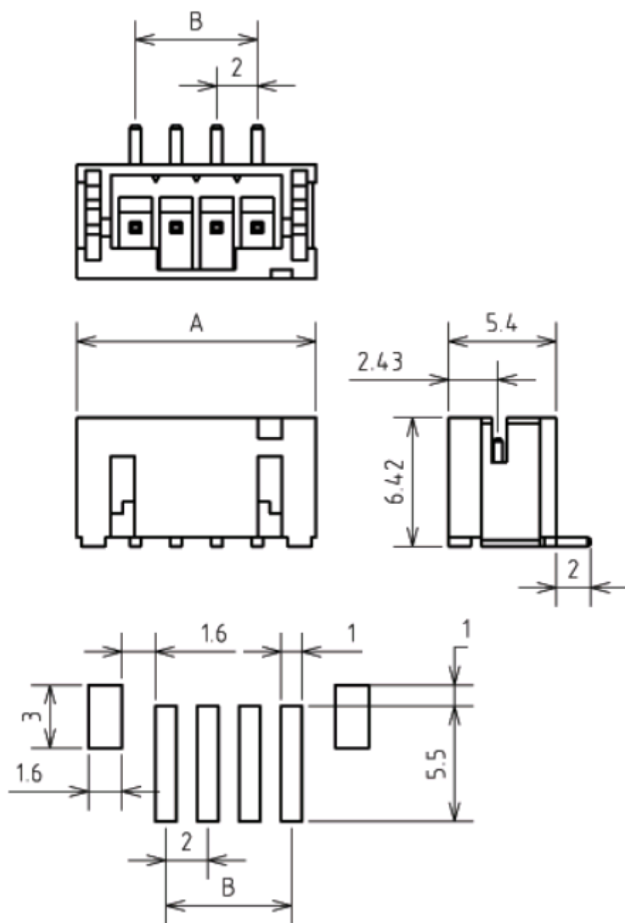
Схема MW-4S
